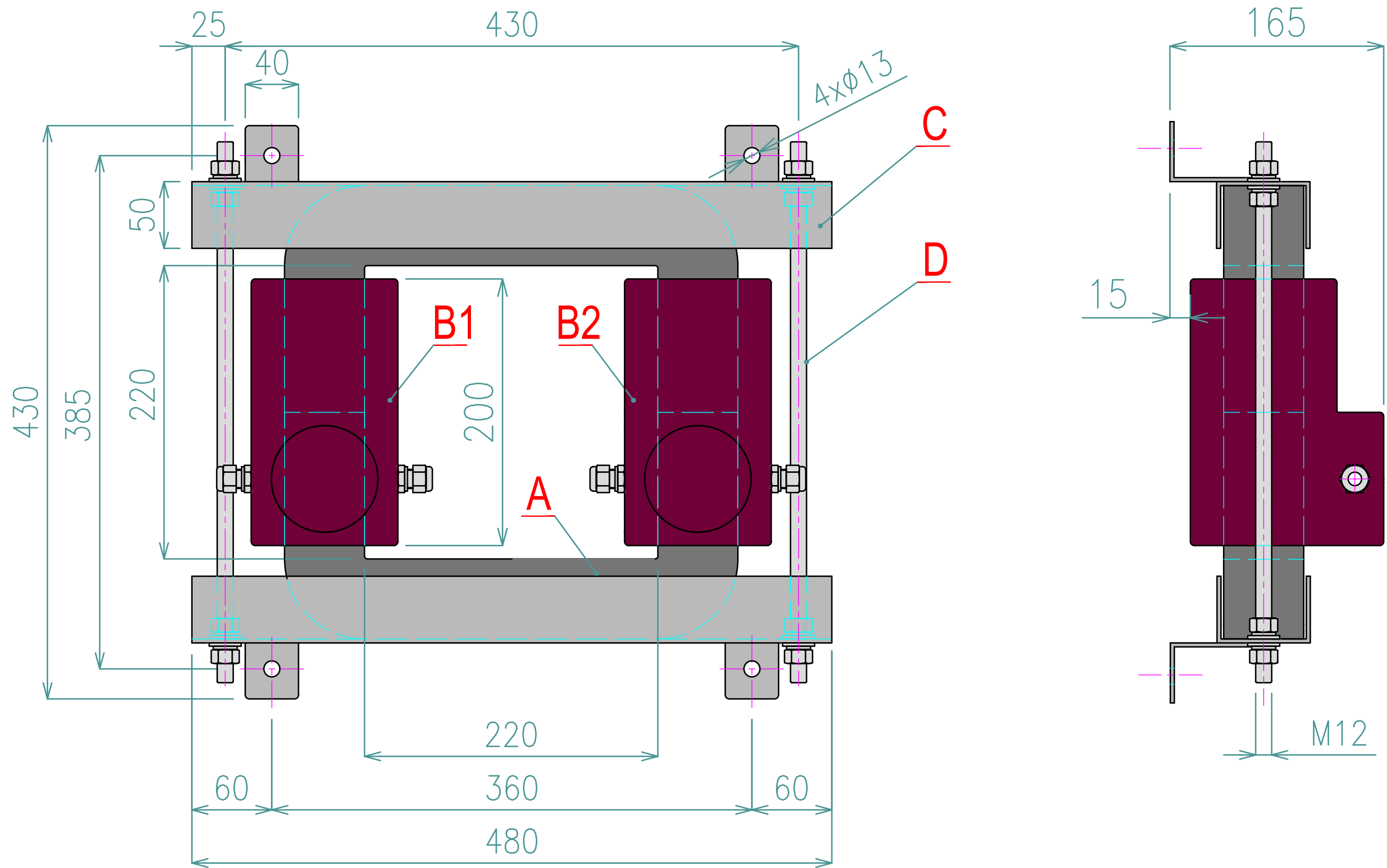
A - magnetický obvod, B1 - sek. vinutí cívka 1, B2 - sek. vinutí cívka 2, C - stahovací konstrukce, D - stahovací svorníky
